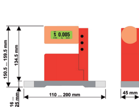
BlueLEVEL with horizontal base mit horizontaler Messbasis
