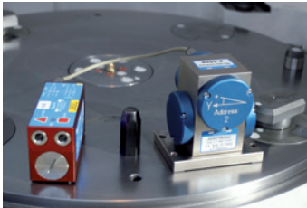
Spindle to round table Spindel zu Rundtisch
