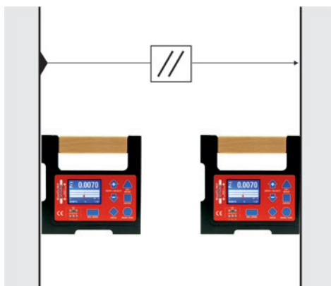
BlueCLINO mit Aluminium-Gehäuse harteloxiert und mit prismatischen Messbasen
